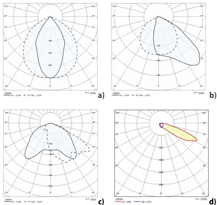
a) ottica simmetrica; b) ottica con asimmetria a 40°; c) ottica con asimmetria a 55°; d) ottica con asimmetria a 65°
